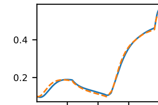
NADH
