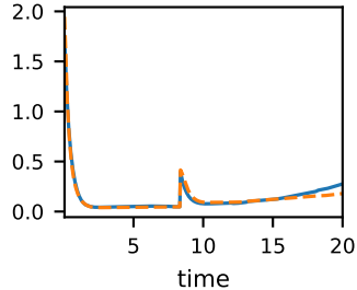
ATP
