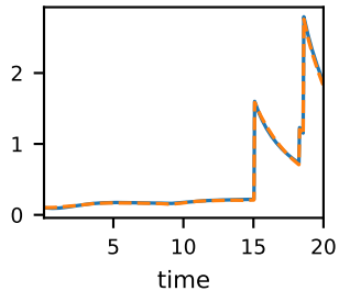
NADH
