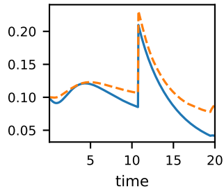
NADH
