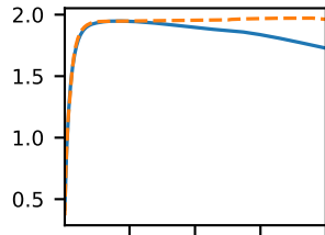
SugarP
