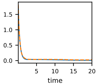
ATP
