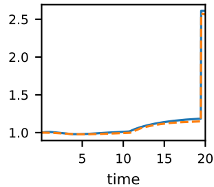
NAD
