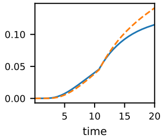
Lac
