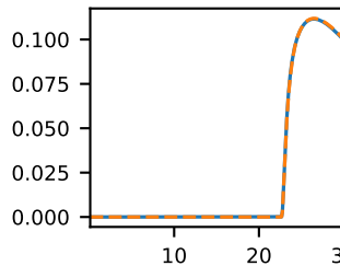
Nuc_C
