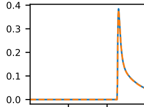
Nuc_C
