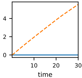
Nuc_C
