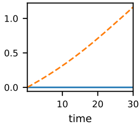
Nuc_C
