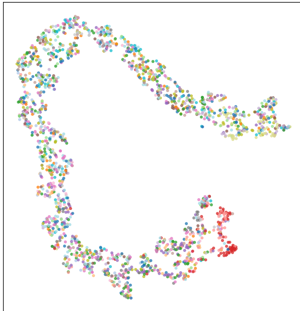
VICReg
