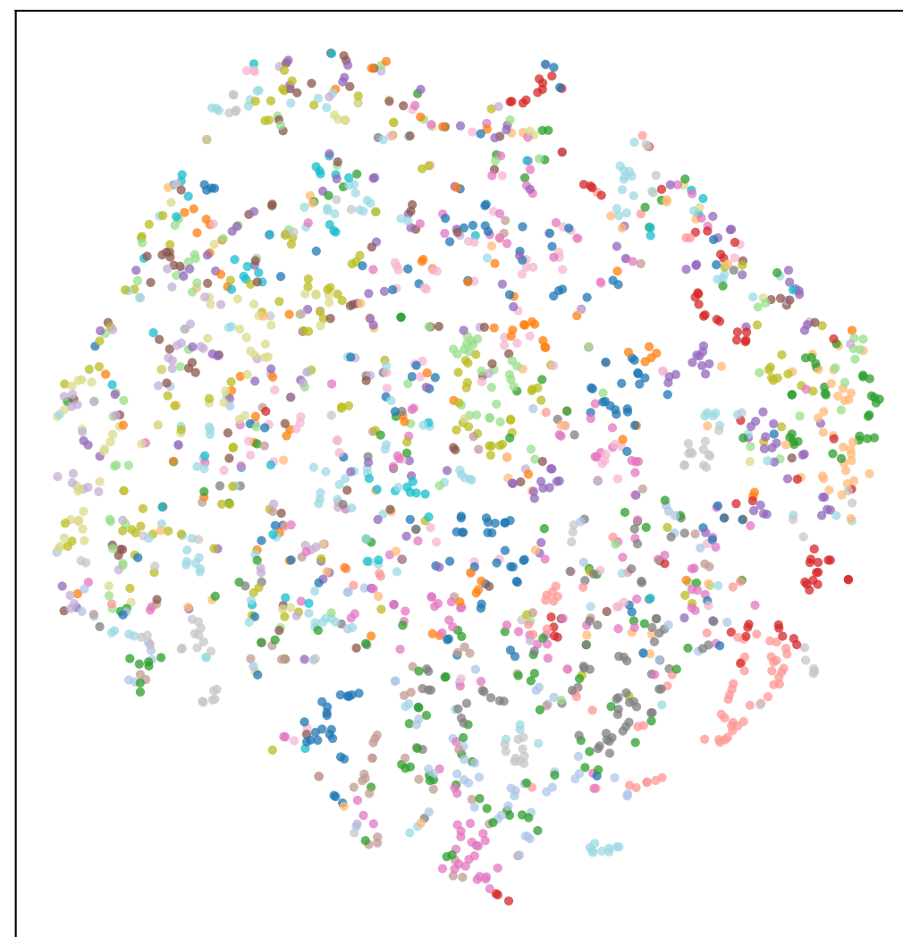
Swav
