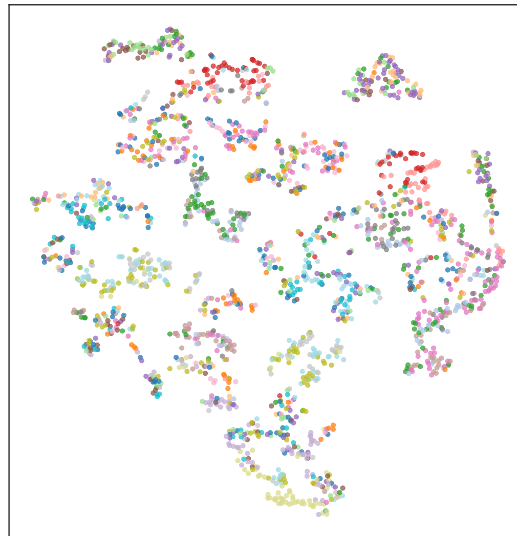
DINO
