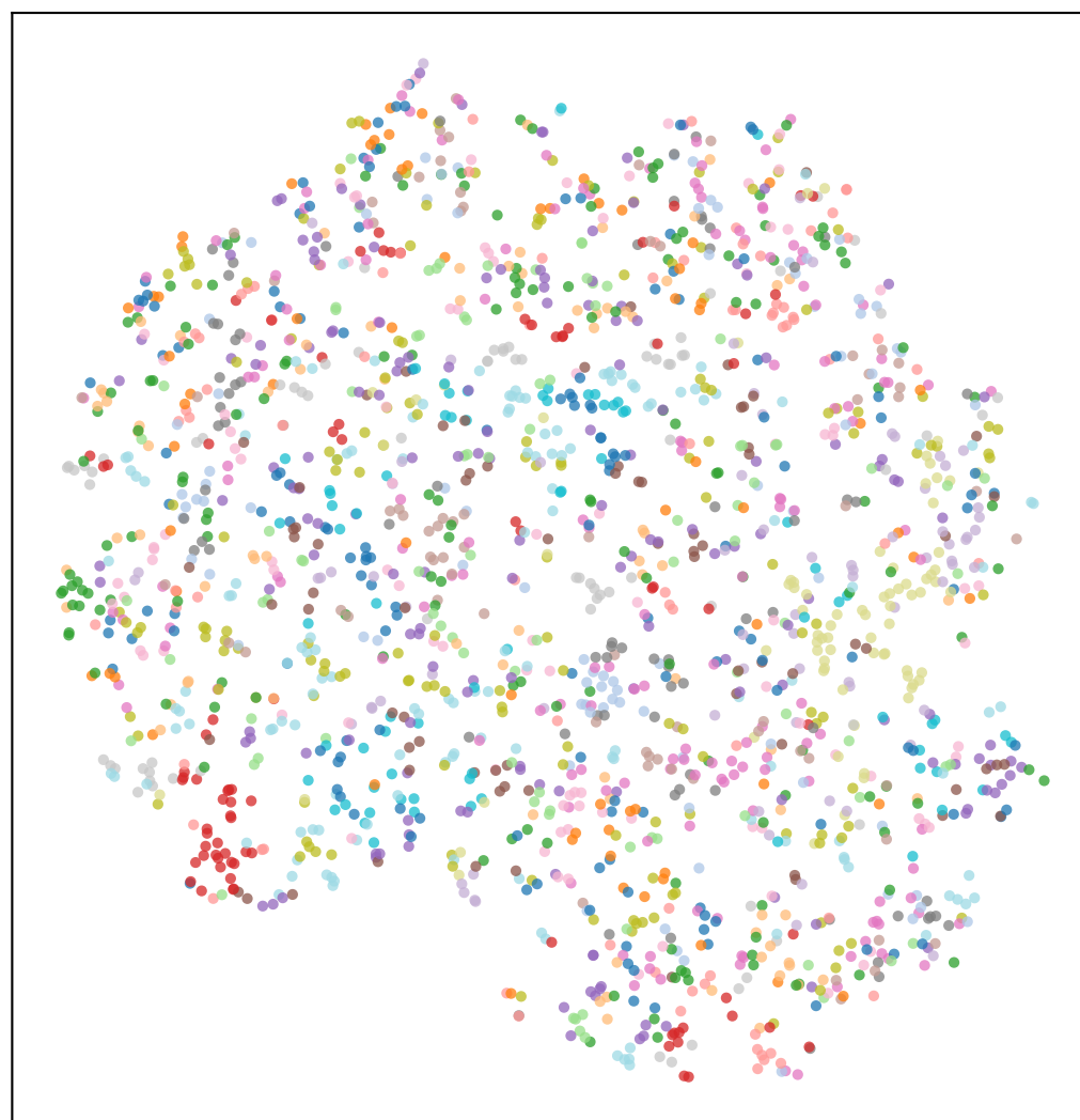
SimSiam
