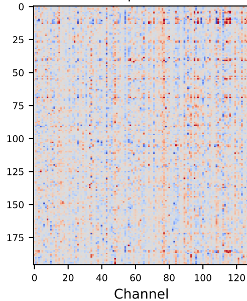
GABA-M1_L Rank=128 | EffRank=87.7
