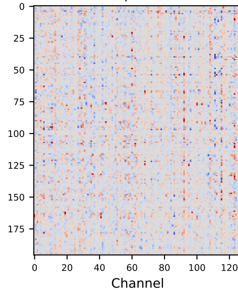
GABA-M2_L Rank=128 | EffRank=88.5
