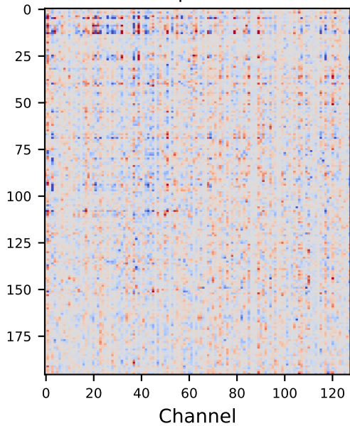
RALA_L Rank=128 | EffRank=80.7
