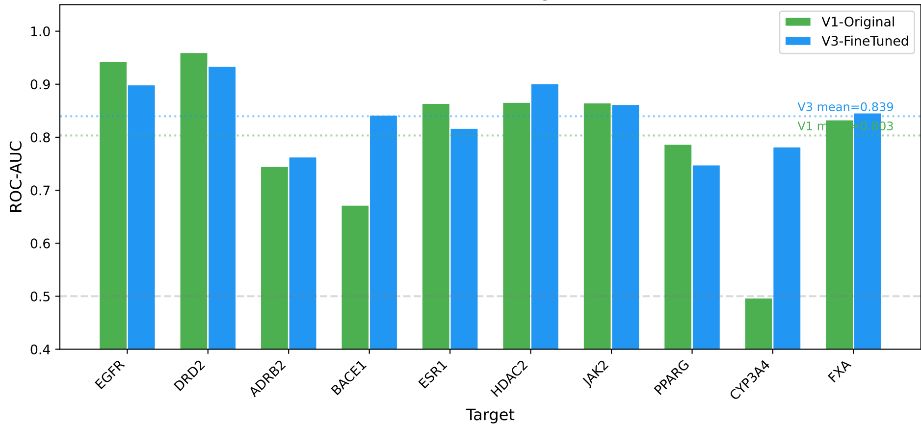
DUD-E Virtual Screening: V1 vs V3
