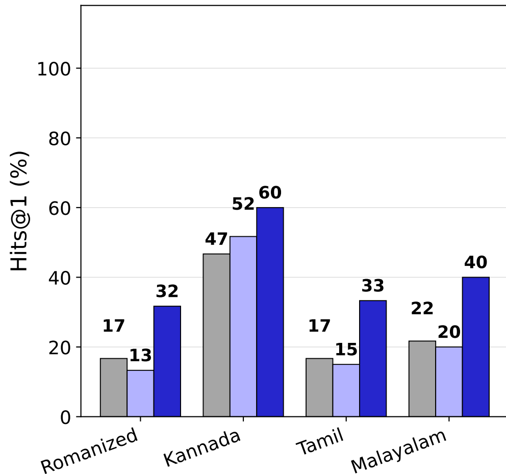
Llama3
