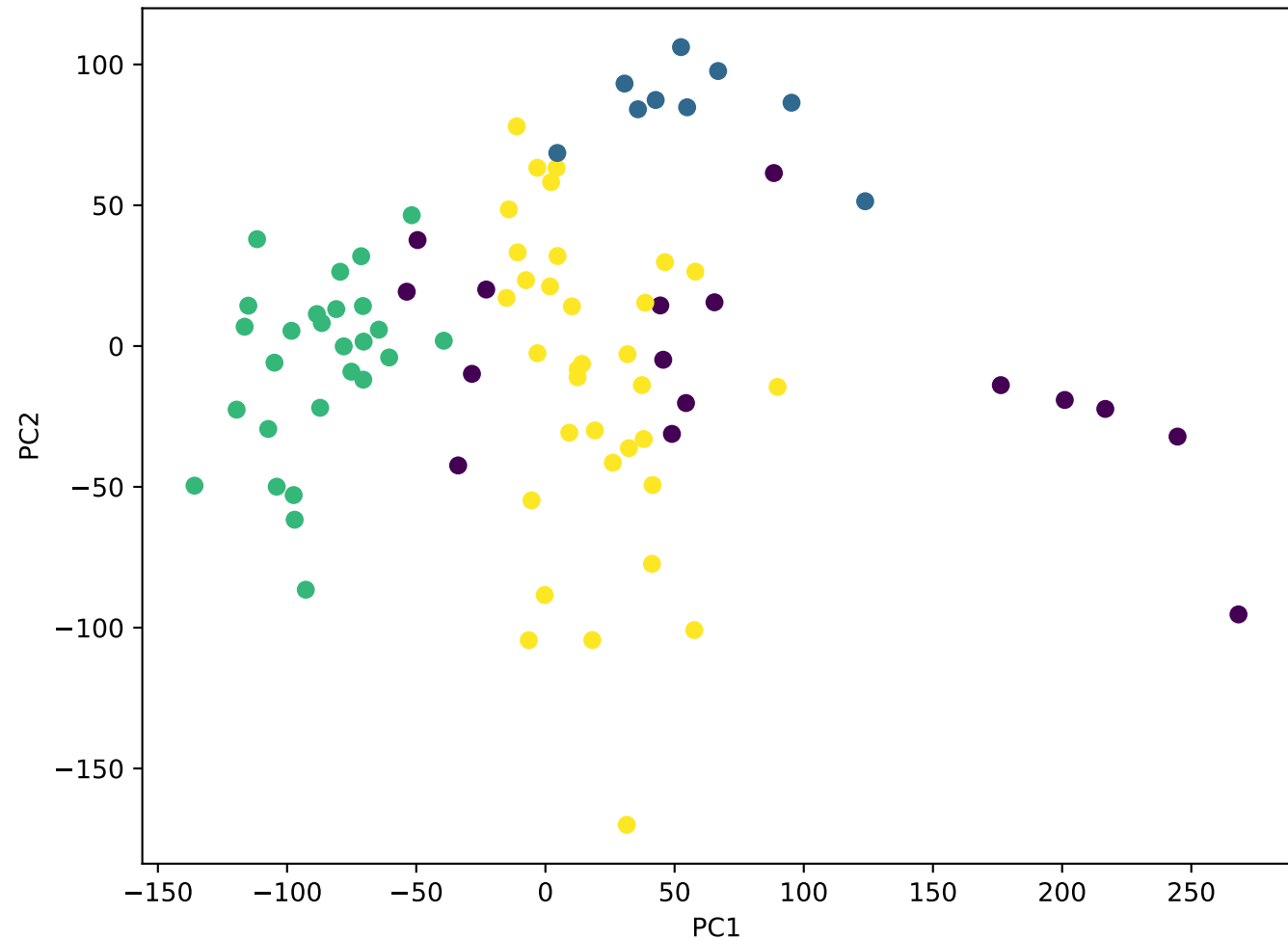
HDBSCAN
