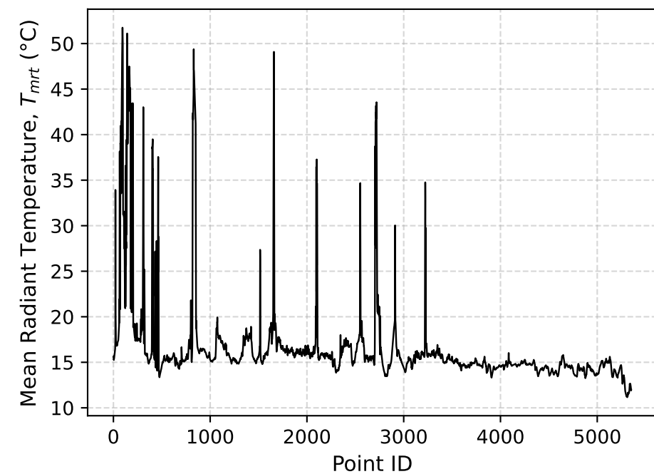
tmrt
