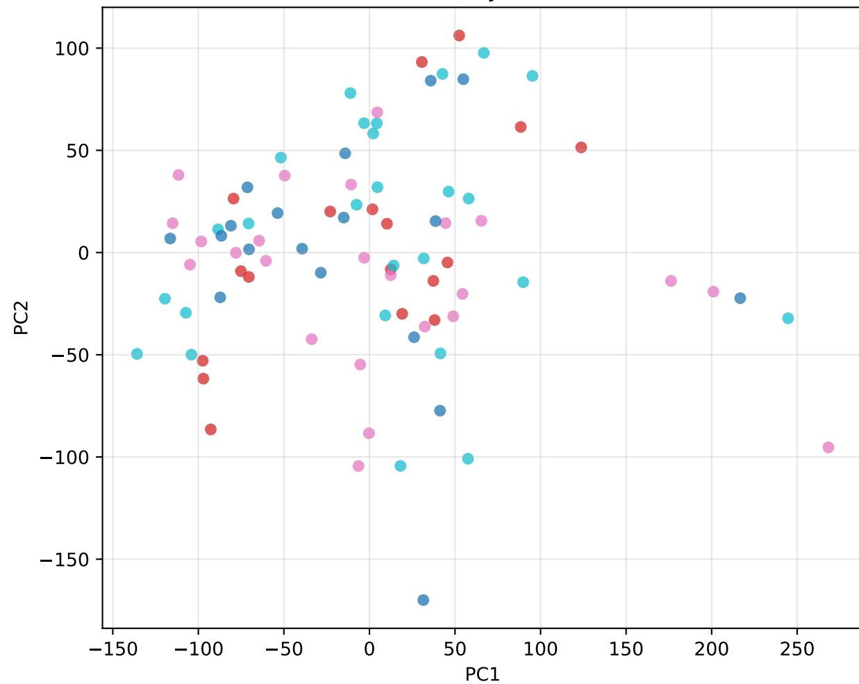
PCA Projection
