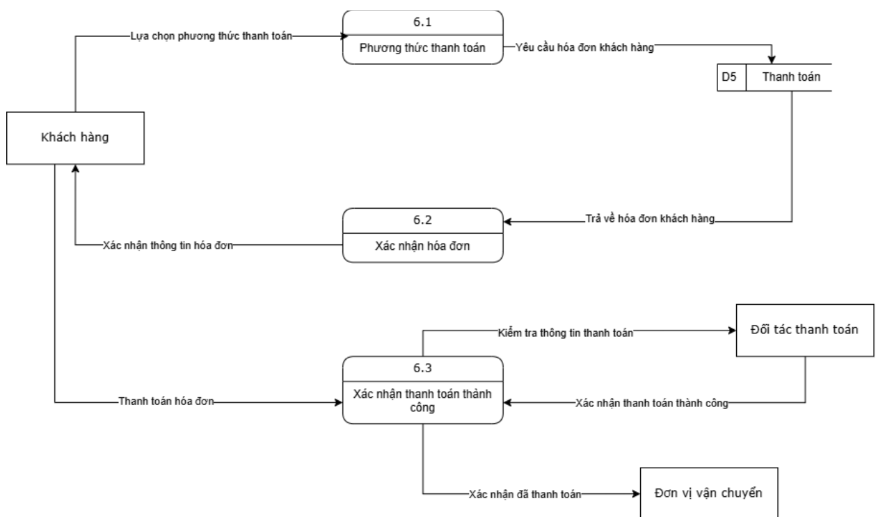
Hình 8: Sơ đồ DFD mức 1 quản lý thanh toán
