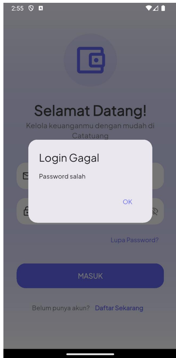
Gambar 2. Password Salah
