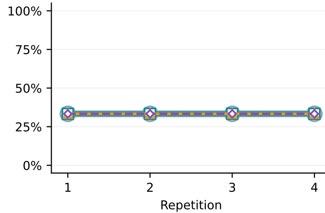
Kimi K3
