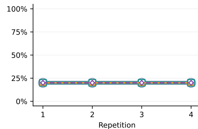
Gemini 3.7 Flash
