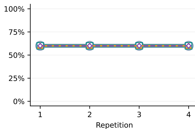
GPT-5 mini
