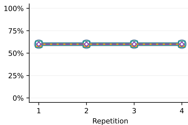
Kimi K3
