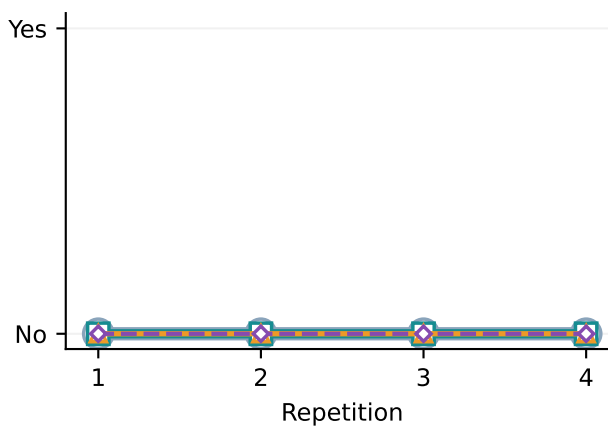
Kimi K3
