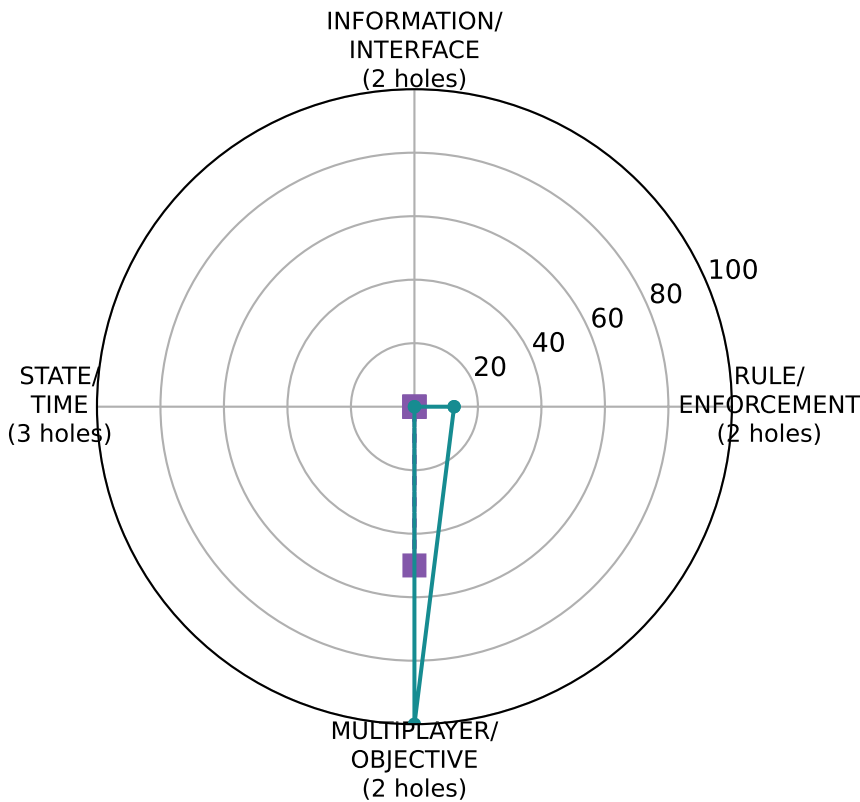
gpt-5
