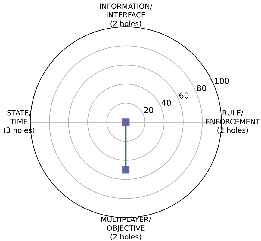
gemini-3.1-pro
