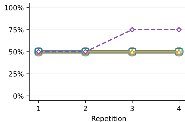
Kimi K3
