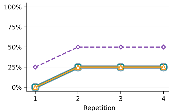
GPT-5 mini
