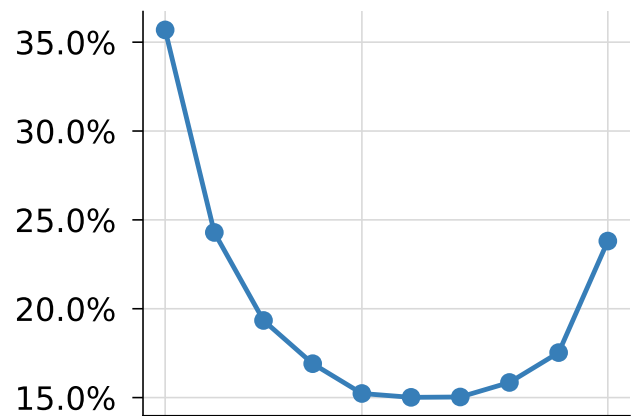
Momentum decile
