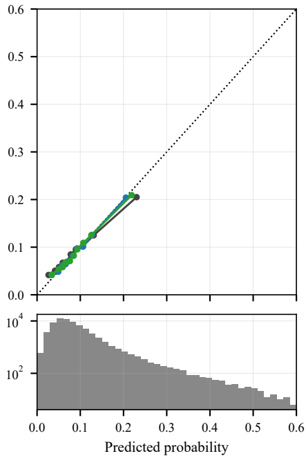
HGB
