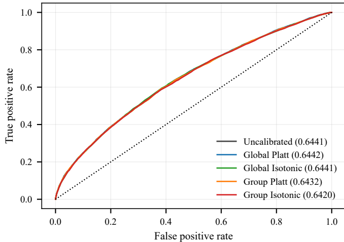
ROC — HGB
