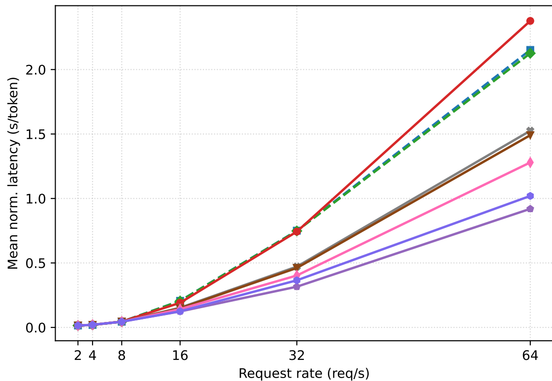
ShareGPT
