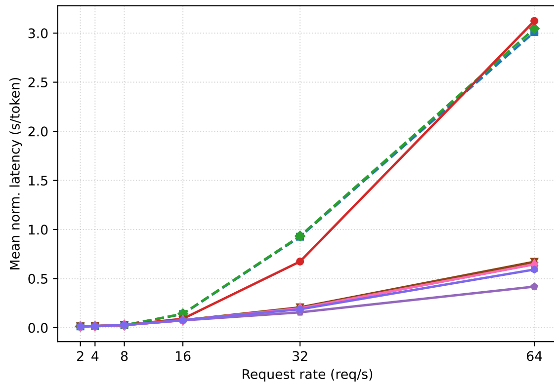
LMSYS-Chat-1M
