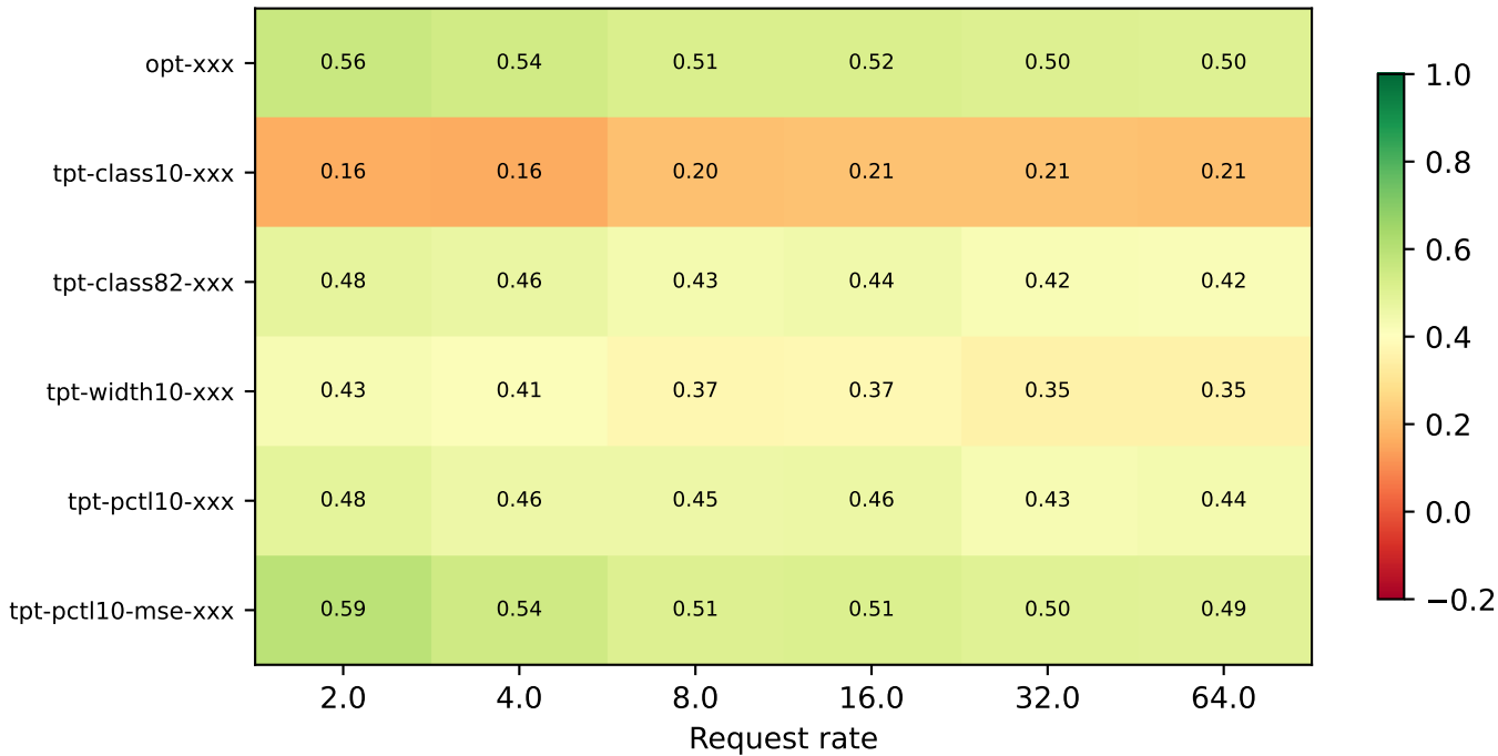
Kendall tau vs SJF -- sharegpt
