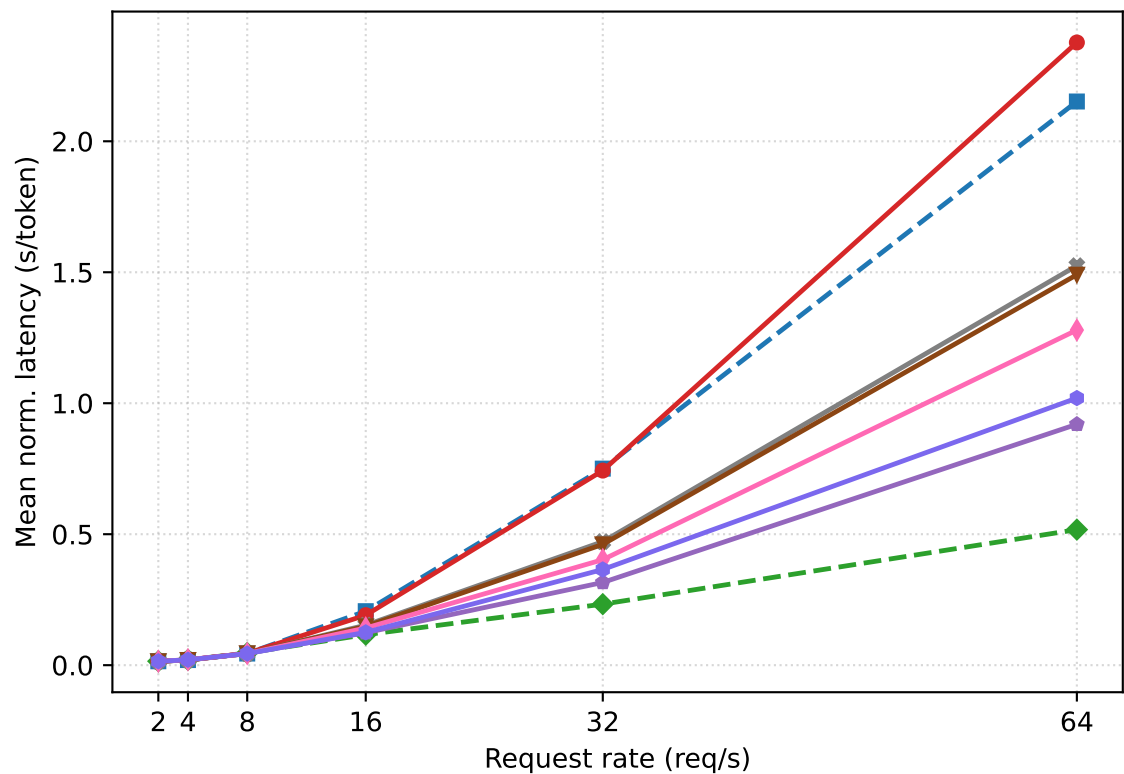
ShareGPT
