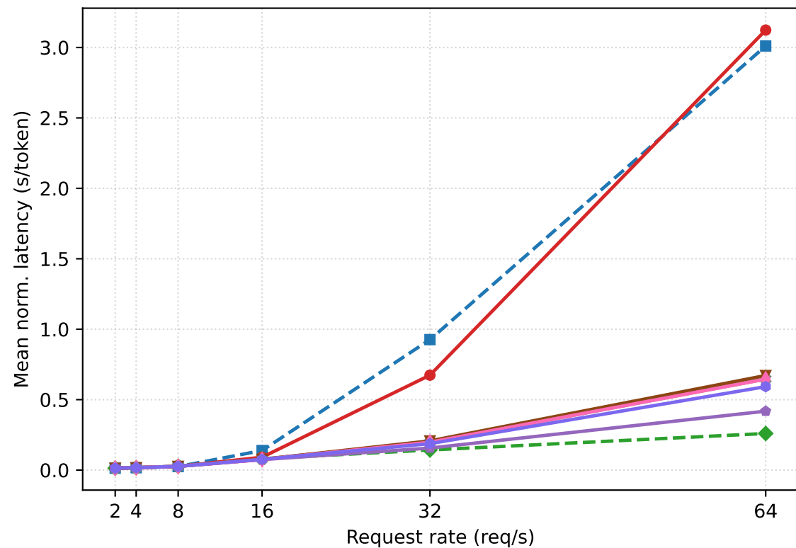
LMSYS-Chat-1M
