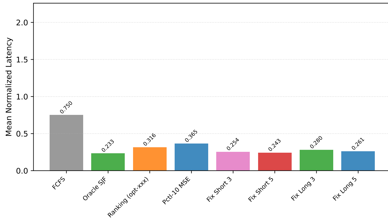
ShareGPT — rate=32
