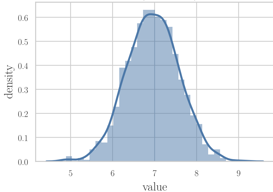
cgpa (skew -0.01)
