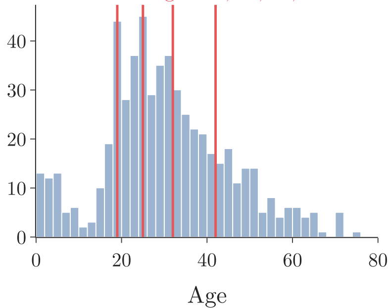
Equal frequency (quantile)
