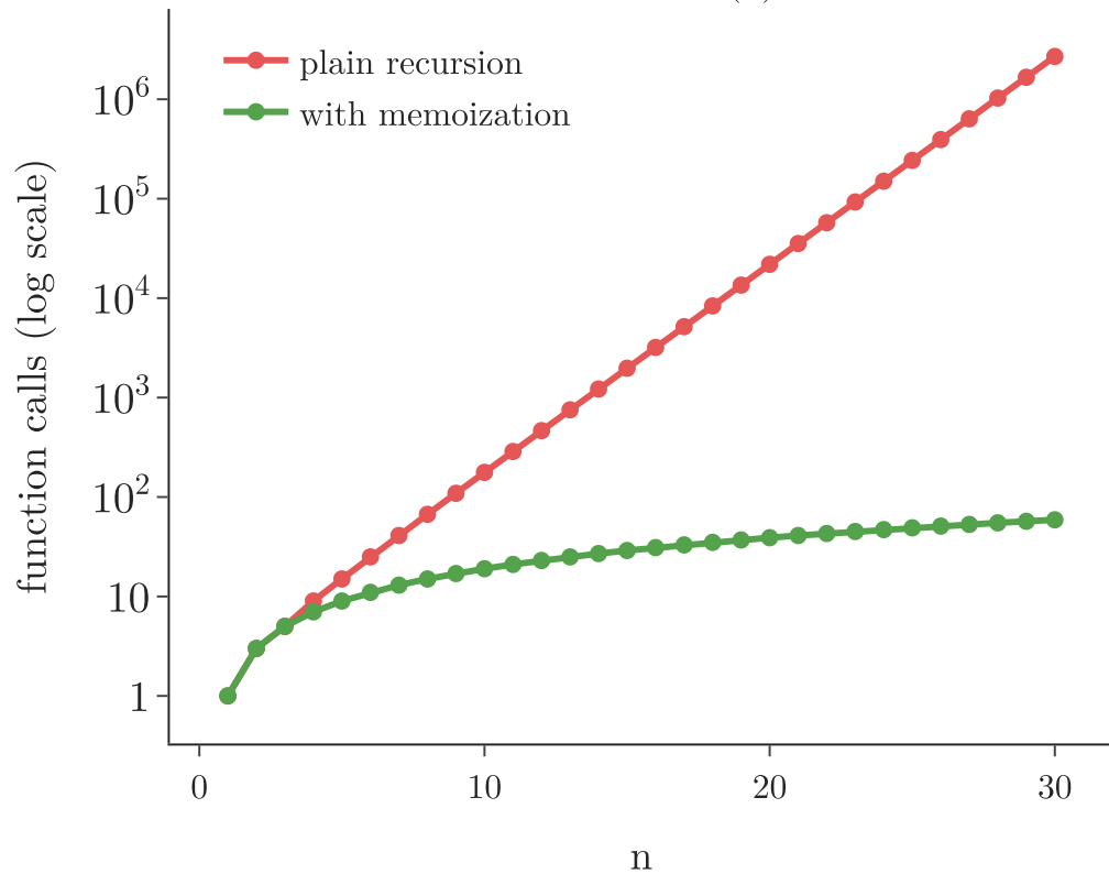
Fibonacci: fib(n)
