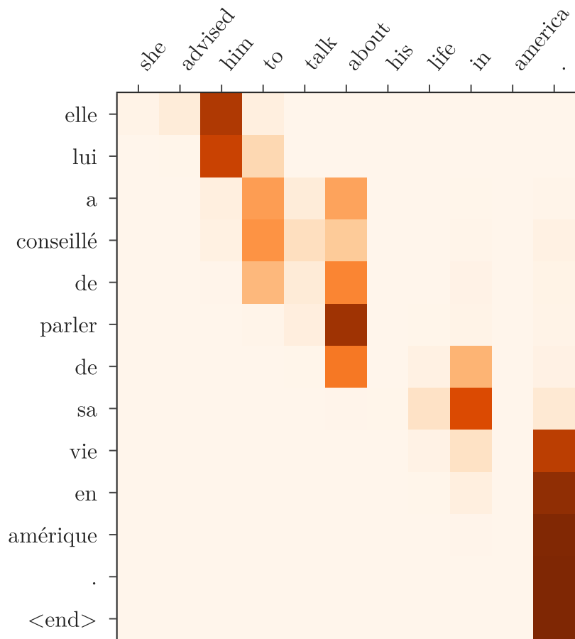
Bahdanau (concat)
