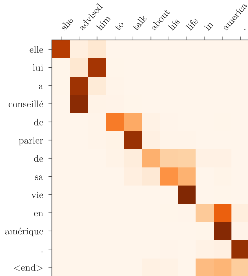
Luong dot
