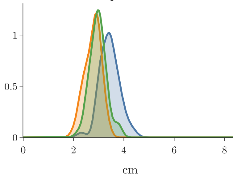
sepal width
