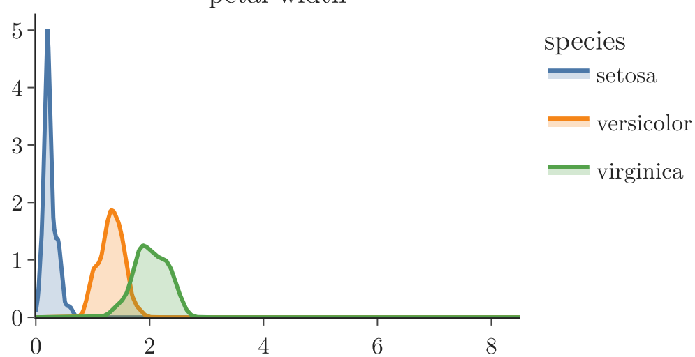
petal width
