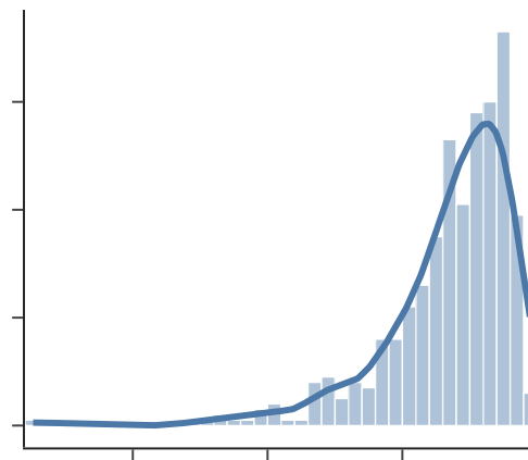
Left skew
