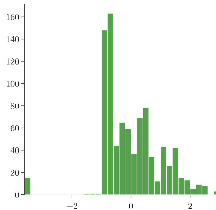
PowerTransformer() skewness -0.04
