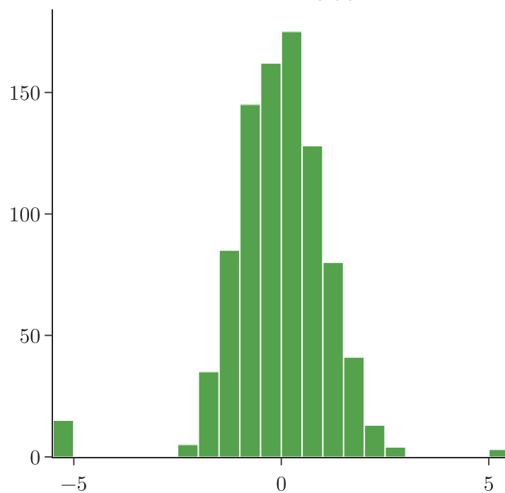
QuantileTransformer(normal) skewness -0.93
