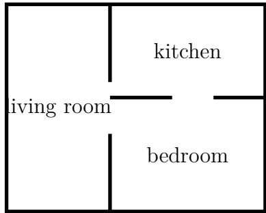
metric map
