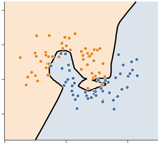
No regularisation
