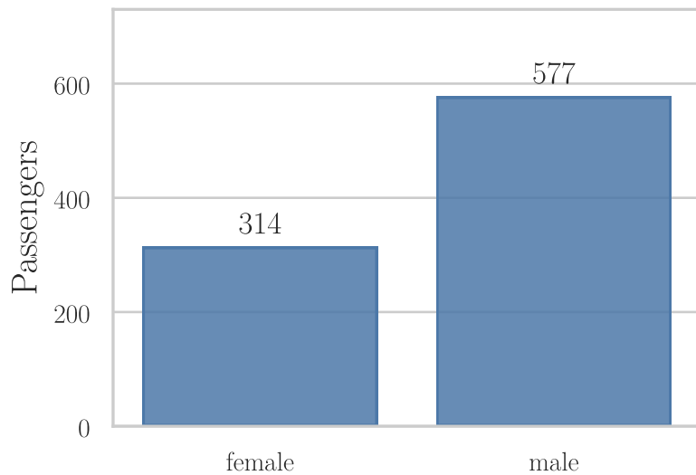
Sex
