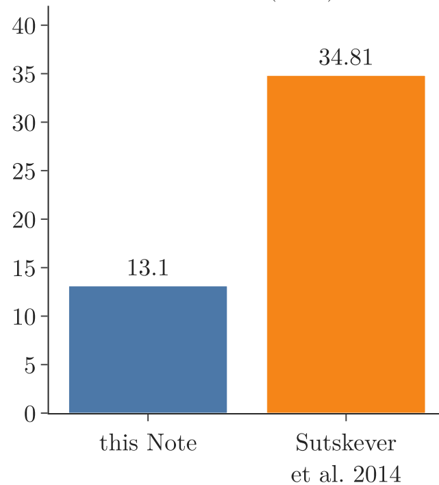
test BLEU (0-100)
