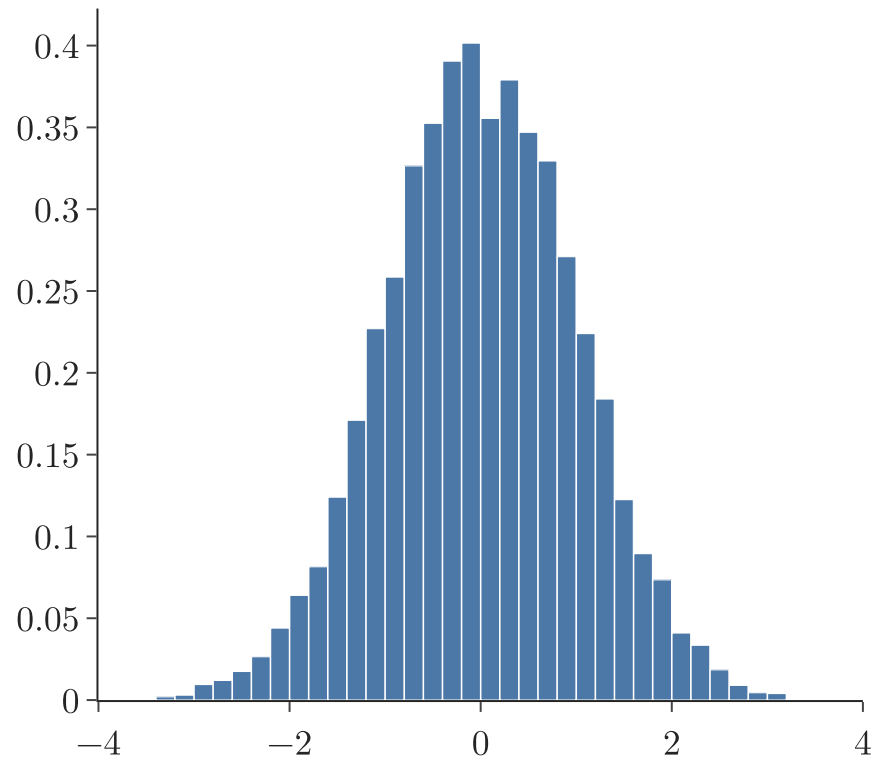
normal: skewness -0.03
