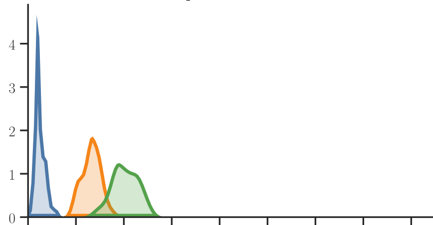
petal width
