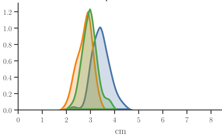
sepal width
