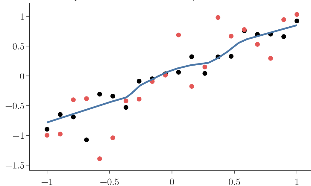
p = 0.2 : train MSE 0.024, test MSE 0.135
