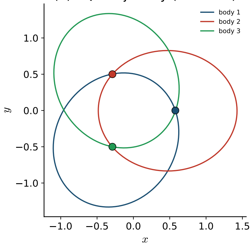
(d) EQ1 trajectory (T=7.715)
