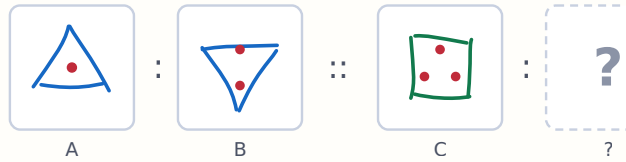
चित्र 33.2 — नियम — 180° घूर्णन तथा एक बिंदु जोड़ना
