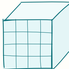
चित्र 38.2 — रंगा घन 4 \times 4 \times 4
