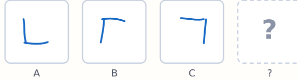
चित्र 33.1 — प्रत्येक चरण में 90° घूर्णन
