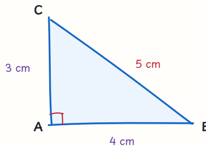
चित्र 16.7 — पाइथागोरस प्रमेय — (कर्ण)^2 = (आधार)^2 + (लंब)^2 , त्रिक (3, 4, 5)
