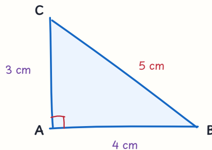
चित्र 16.7 — पाइथागोरस प्रमेय — (\text{कर्ण})^2 = (\text{आधार})^2 + (\text{लंब})^2 , त्रिक (3, 4, 5)
