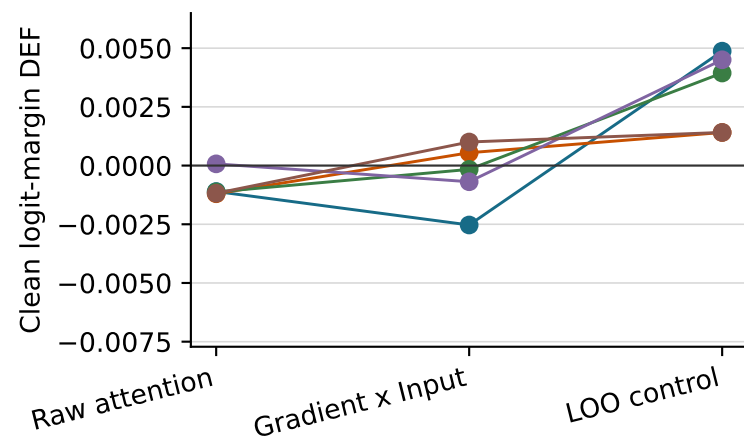
GAT
