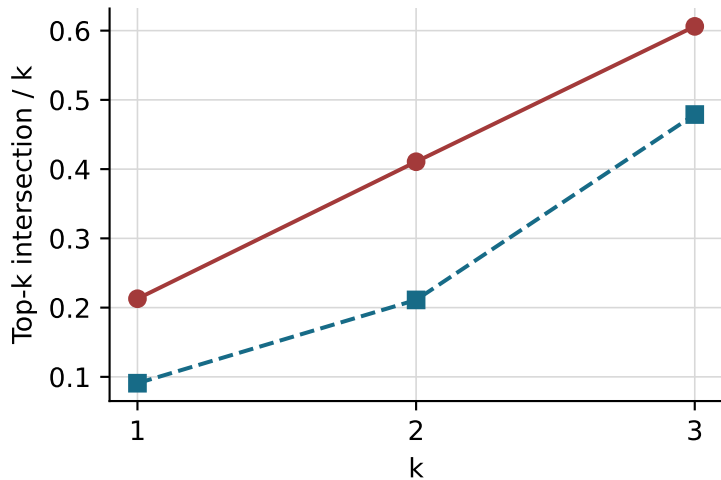
GAT
