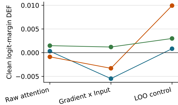
GAT
