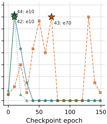
GAT
