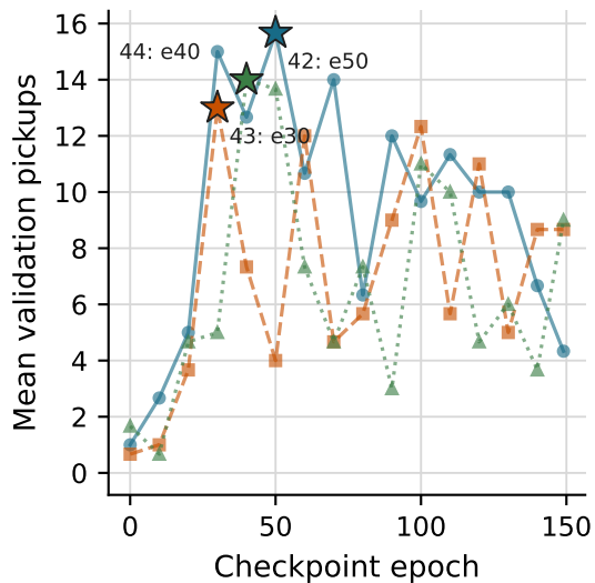
MLP
