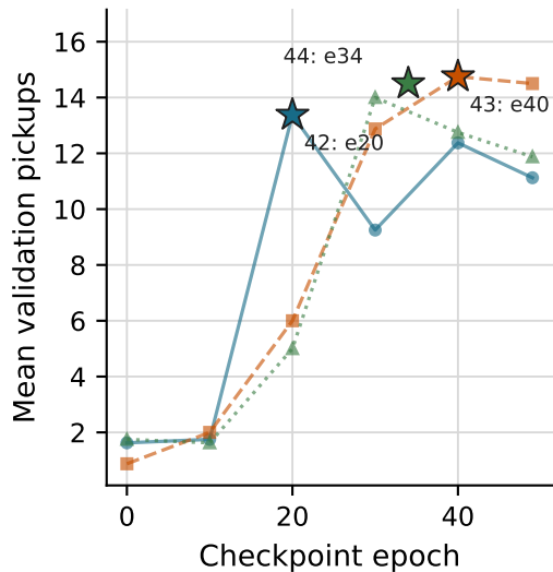
MLP
