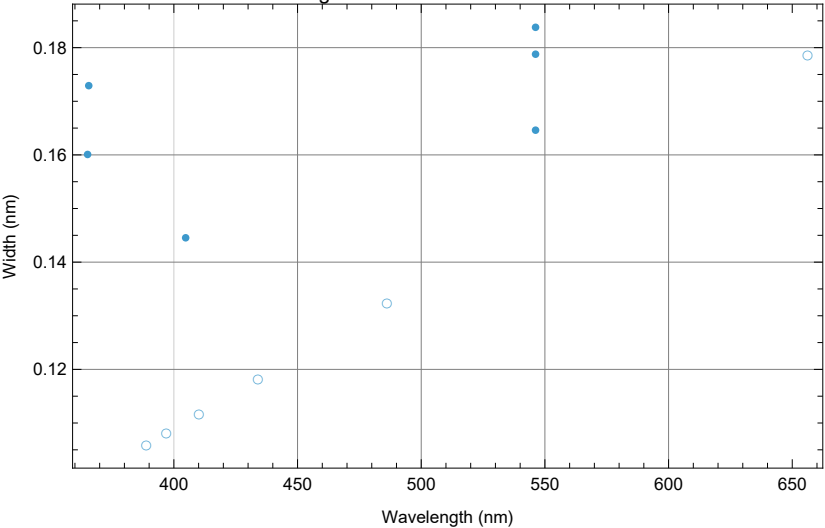
Hg instrumental width estimate
